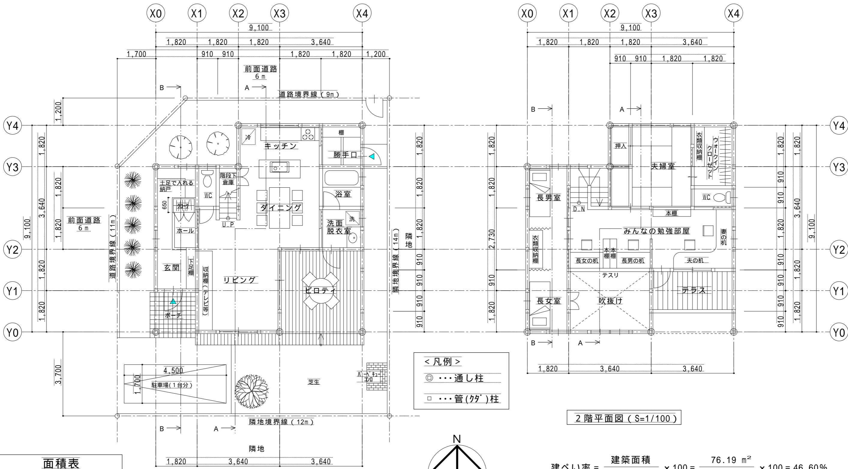
配置図兼1階平面図 (S=1/100)
