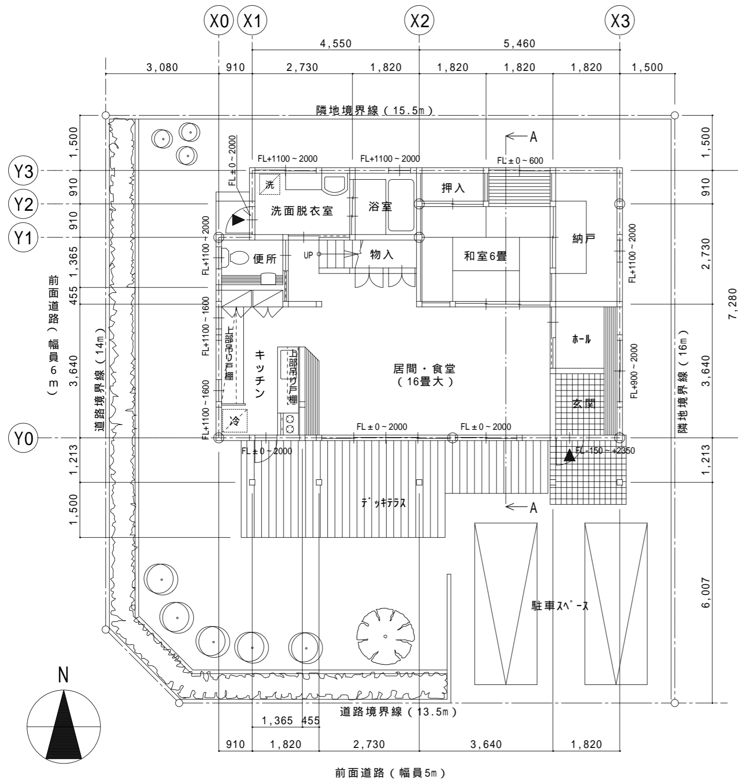
配置図兼 1 階平面図 ( S=1/100 )
